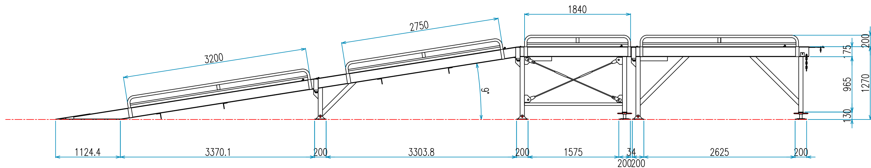
架台1-1 (追加平台)
